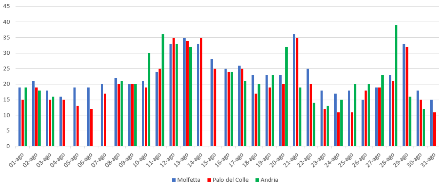
Valori Pm10 nel mese di Agosto
