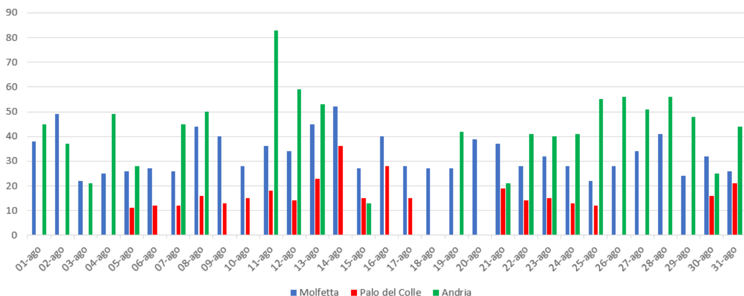
Valori No2 nel mese di Agosto
